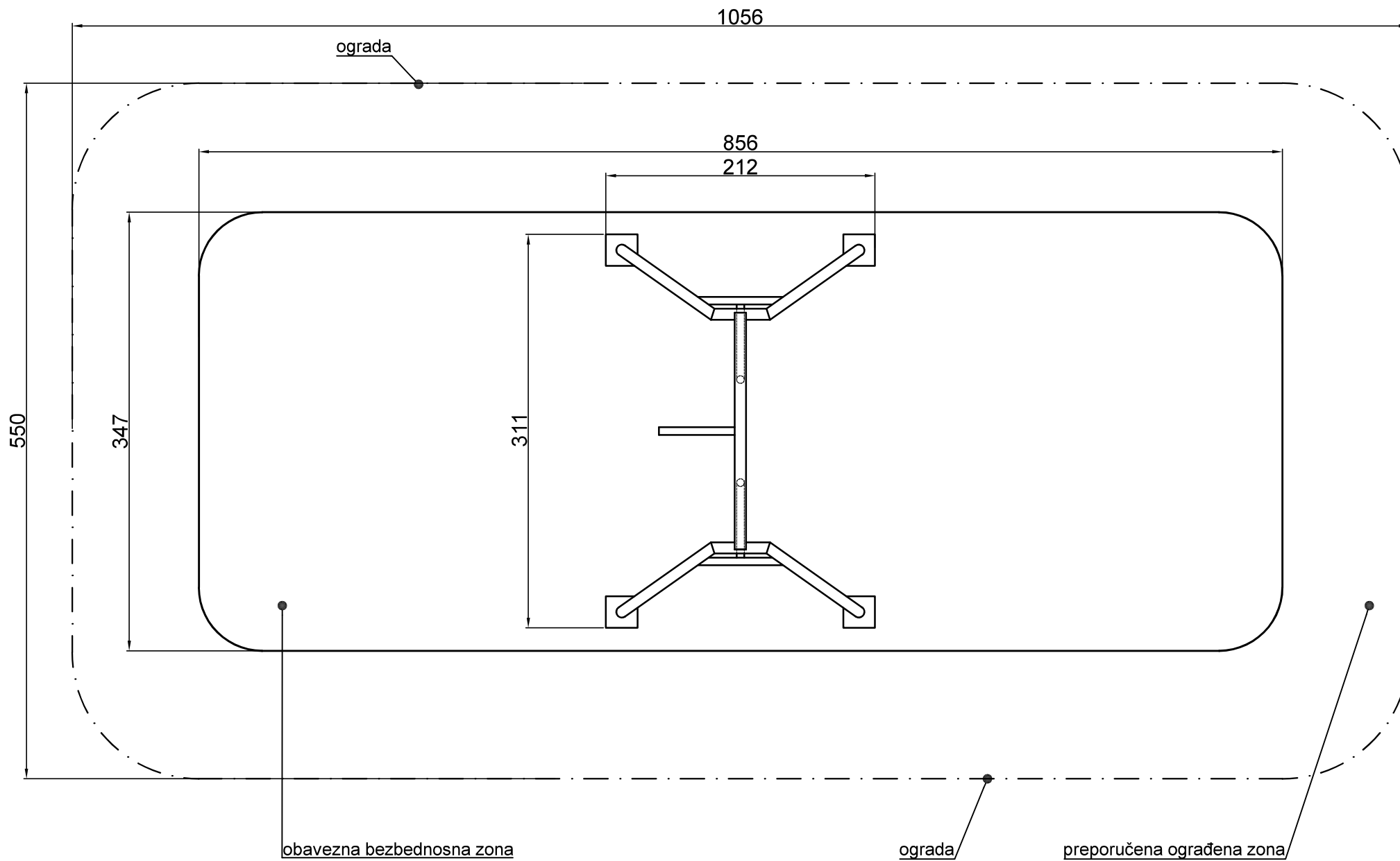
Pogled od gore - Ljuljaška za decu u invalidskim kolicima
